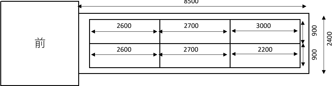
トラック 1台目・2台目（側面図）
