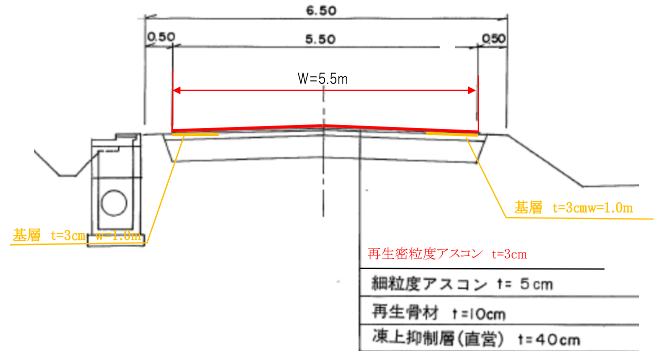
施工図
