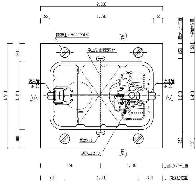
内部平面図 1/25
