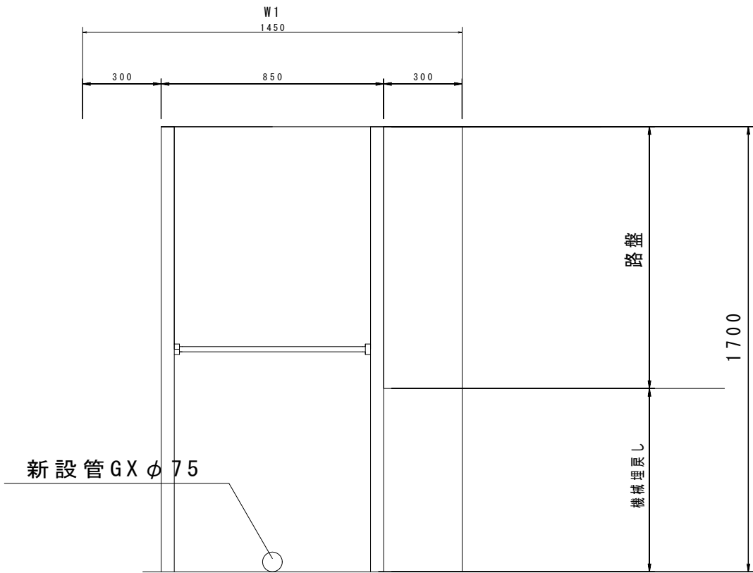
断 面 図 S= 1 : 1 0
