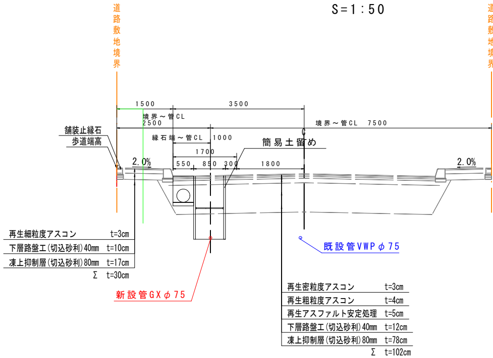
標 準 定 規 図
