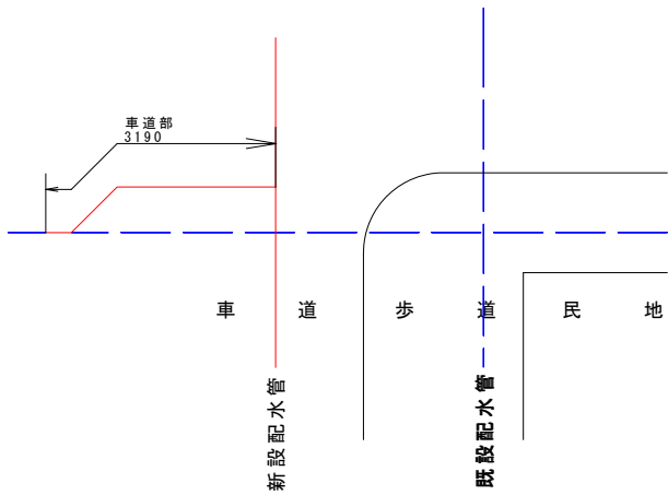
分岐工②④ 平面図 S=1:50
