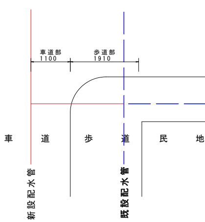
分岐工①③ 平面図 S=1:50
