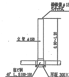
塩ビ点検槽φ100-150
